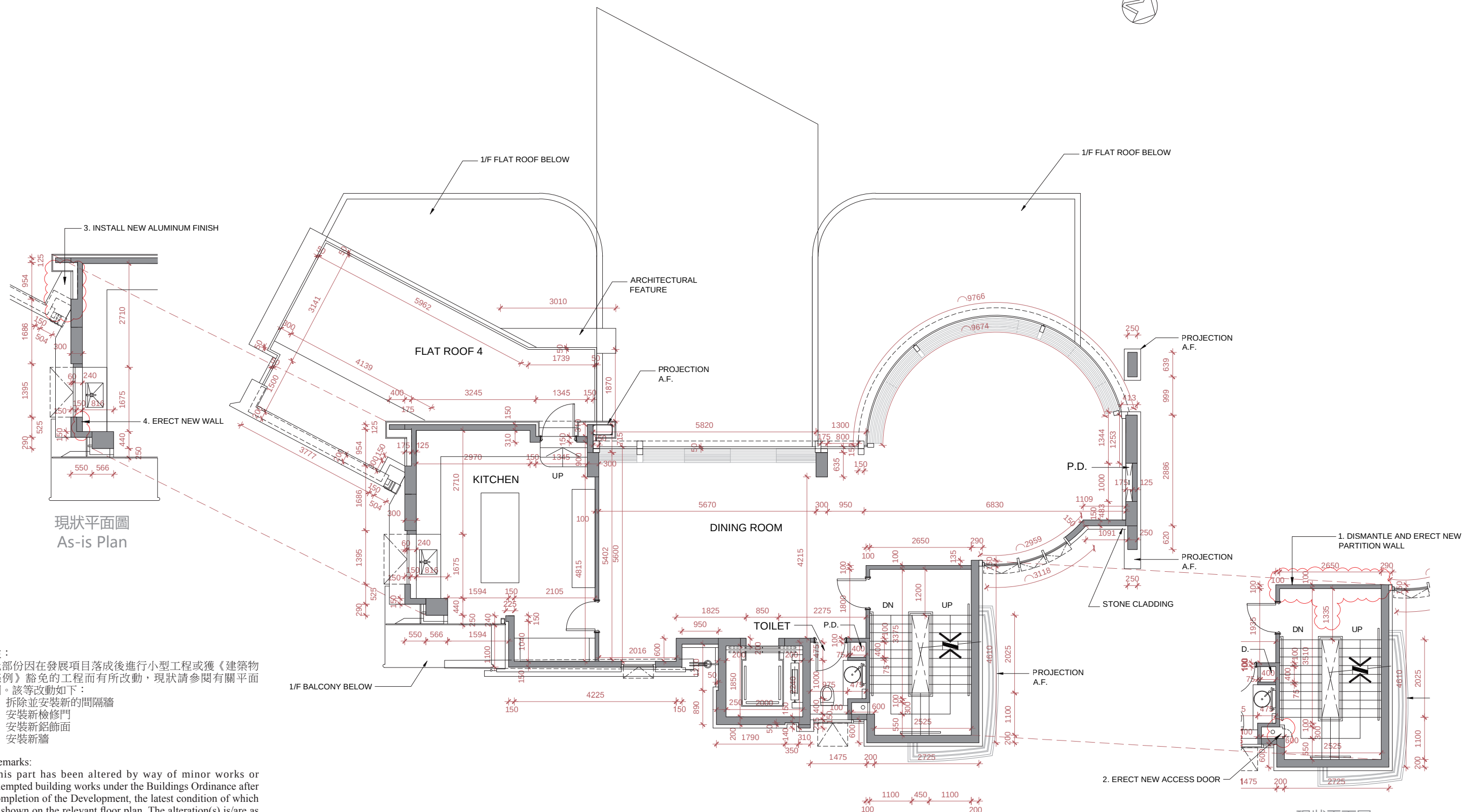
洋房2 2樓樓面平面圖 House 2 2/F Floor Plan
